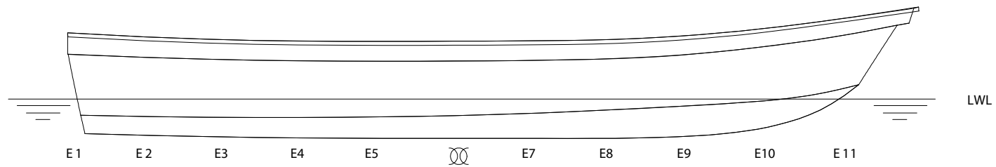
VISTA LATERAL
