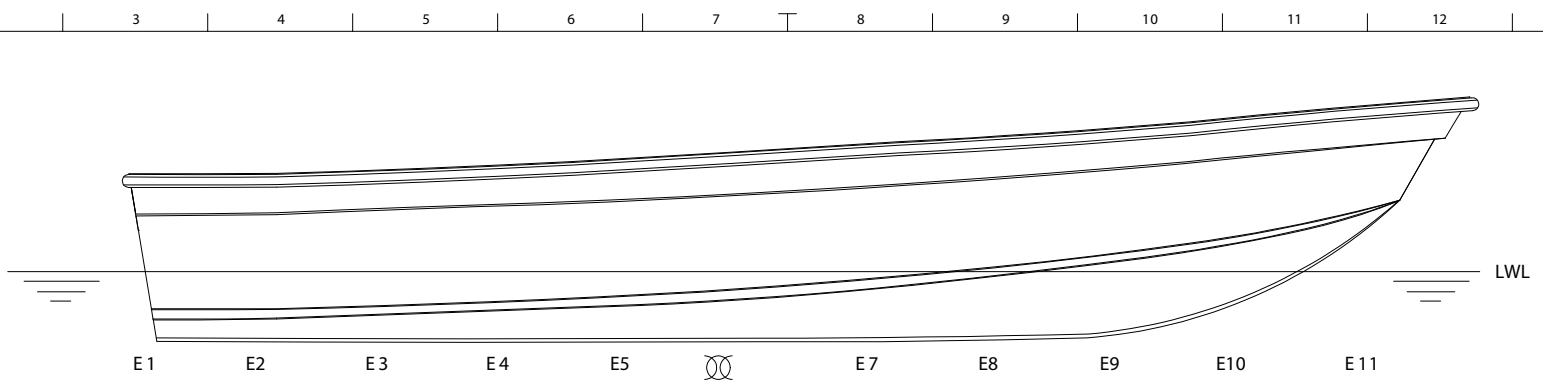
VISTA PERFIL
