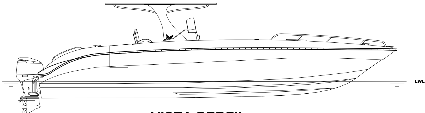
VISTA PERFIL
